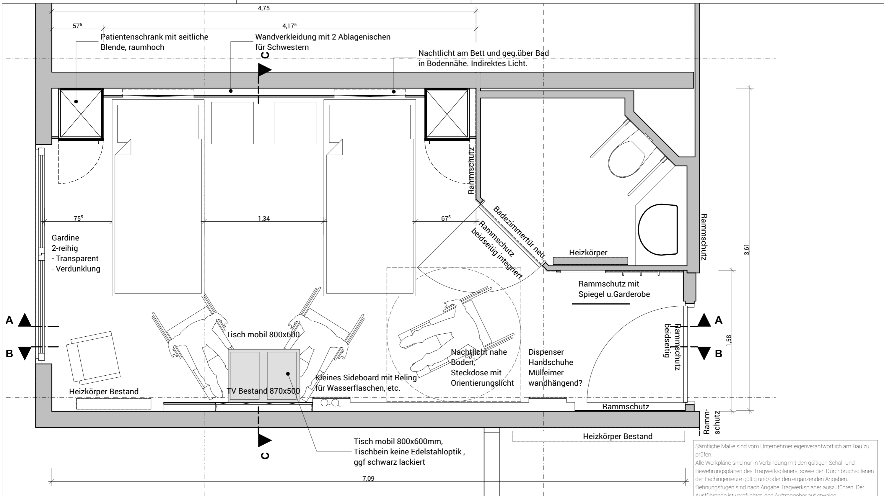
Grundriss Musterzimmer
