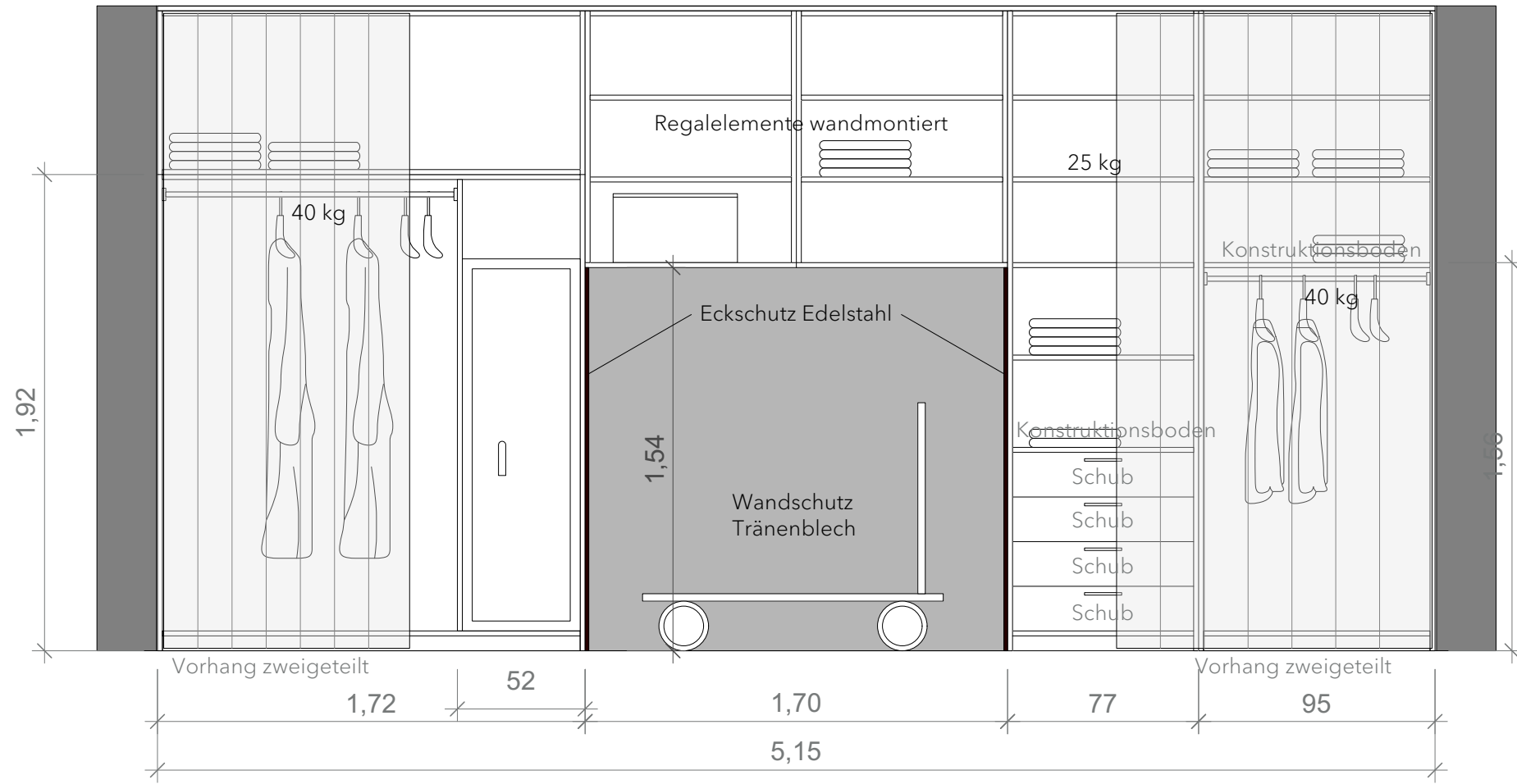
Schrankseiten mit durchgehender Lochreihe für verstellbare Einlegeböden
