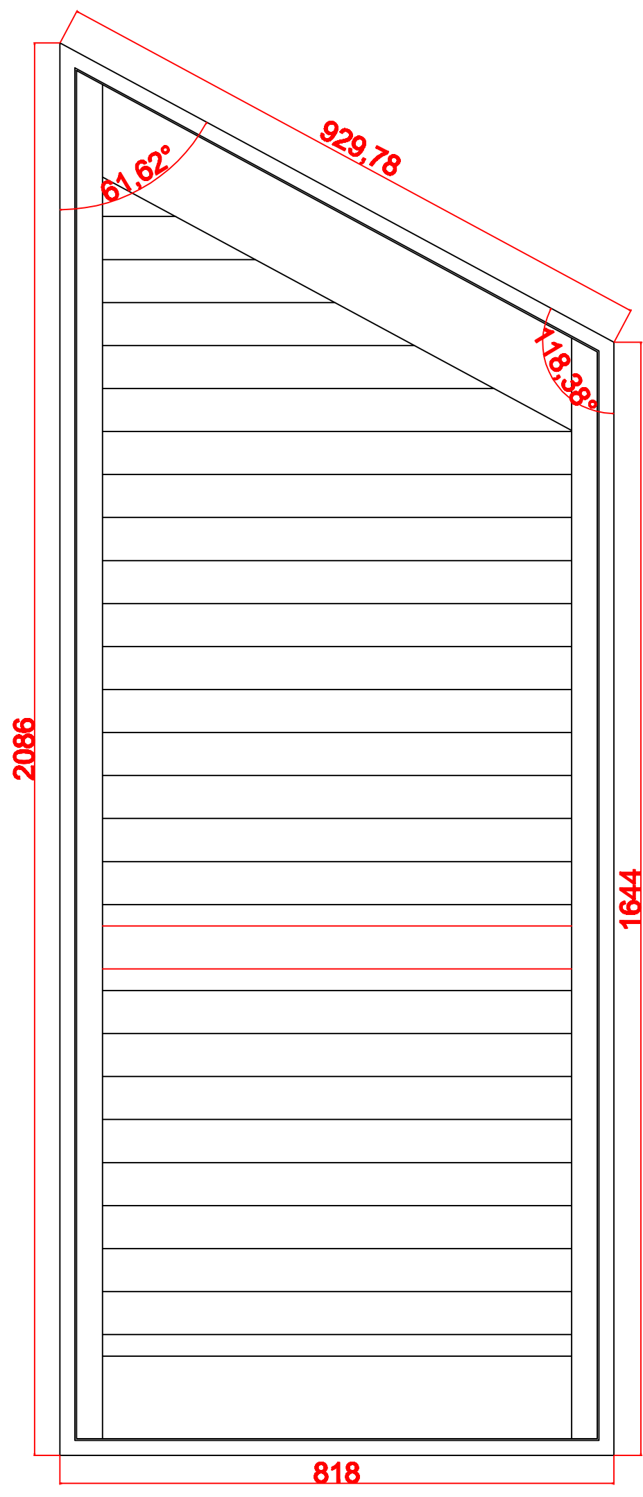
HP-4240-1-L Extra louvres *2
