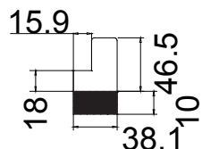
Plain L Frame 46mm(+10)
