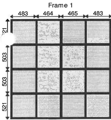
1-1895x2048 Window No: 1 9005 Black - Matt
