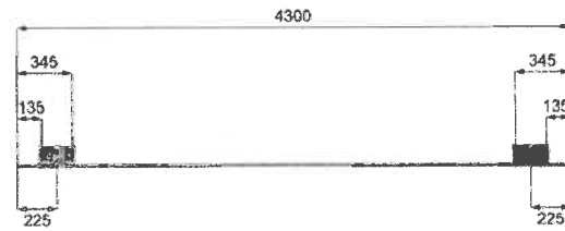
Konsolenplan
