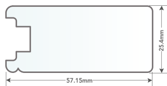
57mm Butt Stile
