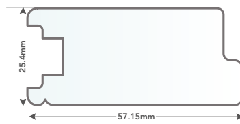
57mm Rebate Stile
