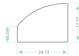
Deco Insert Batten
