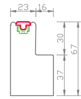
67mm F/F L-Frame
