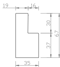
67mm Plain L-Frame
