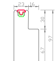
97mm F/F L-Frame
