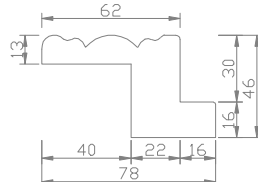
Deco Z-Frame (Z-60/66)
