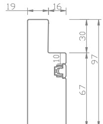
97mm S/F L-Frame
