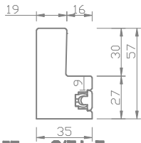
57mm S/F L-Frame
