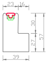
57mm F/F L-Frame
