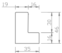
47mm Plain L-Frame
