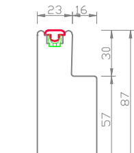
87mm F/F L-Frame
