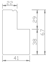
67mm Bead L-Frame
