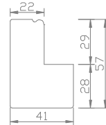
57mm Bead L-Frame
