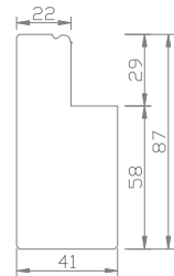
87mm Bead L-Frame
