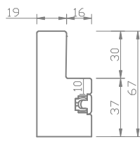
67mm S/F L-Frame
