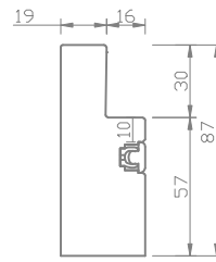
87mm S/F L-Frame
