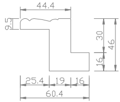
Z-Fine Frame (Z45)
