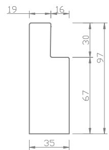
97mm Plain L-Frame
