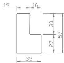
57mm Plain L-Frame
