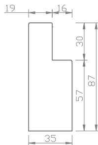
Pv 87mm Plain L-Frame
