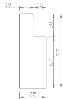
Pv 97mm Plain L-Frame
