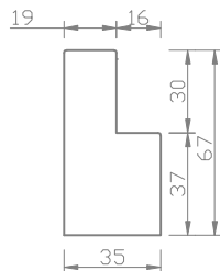
Pv 67mm Plain L-Frame
