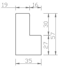
Pv 57mm Plain L-Frame
