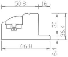
Pv Deco L-Frame
